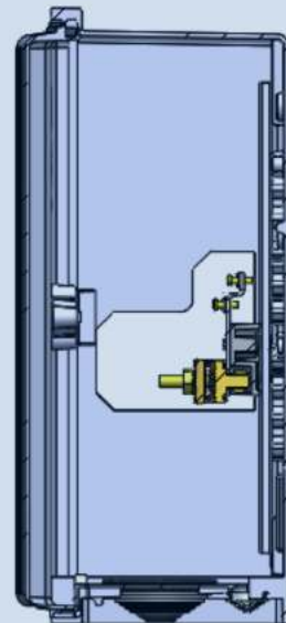
COUPE A-A ECHELLE 1 : 7
