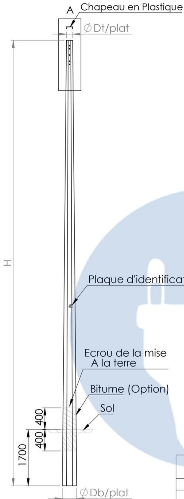
ECHELLE 1 : 50
