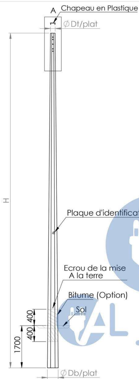
ECHELLE 1 : 50
